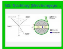
Q2: Atomphysik
